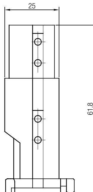
320105-001 Unión mecánica
