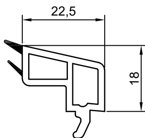
560510-474 Junquillo 22.5 Blanco 560510-174 Junquillo 22.5 Beige 560510-275 Junquillo 22.5 Clay
