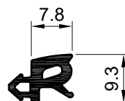
865022-001 Junta de acristalar No. 68
