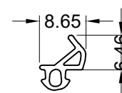
330101-001 Junta de hoja
