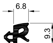
865012-001 Junta de acristalar No. 67
