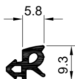
865002-010 Junta de acristalar No. 66
