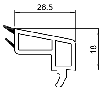
560620-376 Junquillo 26.5 mm Blanco 560620-051 Junquillo 26.5 mm Beige 560620-056 Junquillo 26.5 mm Clay
