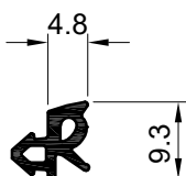
864992-010 Junta de acristalar No. 65
