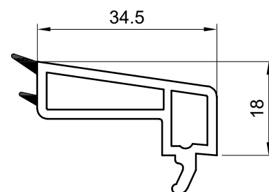
561530-376 Junquillo 34.5 mm Blanco 561530-174 Junquillo 34.5 mm Beige 561530-275 Junquillo 34.5 mm Clay
