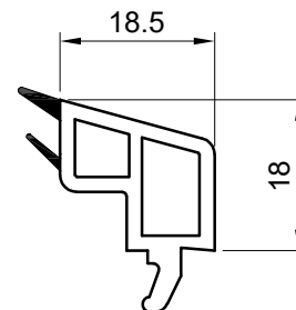
560610-376 Junquillo 18.5 mm blanco 560610-174 Junquillo 18.5 mm beige 560610-275 Junquillo 18.5 mm clay
