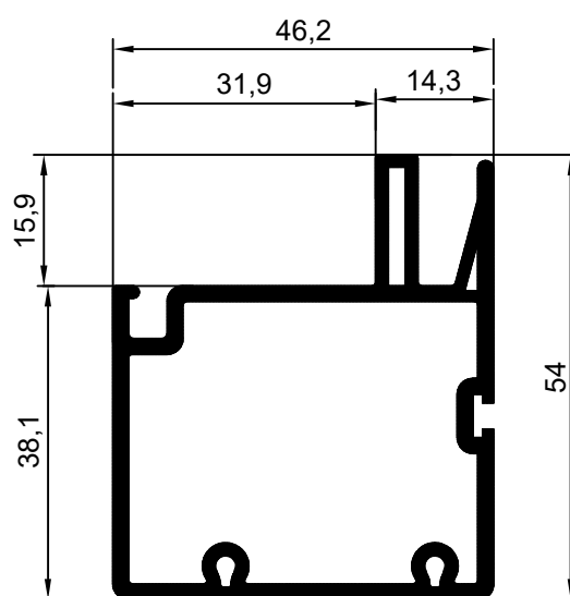
201602-231 Travesaño blanco 201602-233 Travesaño beige 201602-236 Travesaño clay
