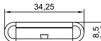
600526-001 Tapa de desagüe Blanco 600526-003 Tapa de desagüe Beige 600526-006 Tapa de desagüe Clay
