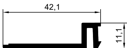
201608-351 Clip Anti elevación 1.5" blanco 201608-353 Clip Anti elevación 1.5" beige 201608-356 Clip Anti elevación 1.5" clay
