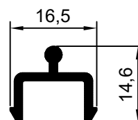
201607-301 Riel de Mosquitero blanco 201607-303 Riel de Mosquitero beige 201607-306 Riel de Mosquitero clay
