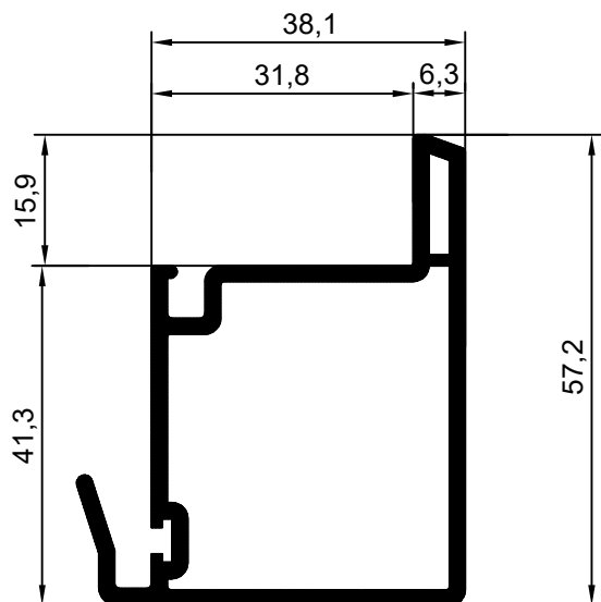
201604-231 Hoja Traslape blanco 201604-233 Hoja Traslape beige 201604-236 Hoja Traslape clay
