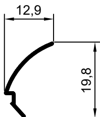
201609-301 Junquillo p/cristal doble blanco 201609-303 Junquillo p/cristal doble beige 201609-306 Junquillo p/cristal doble clay
