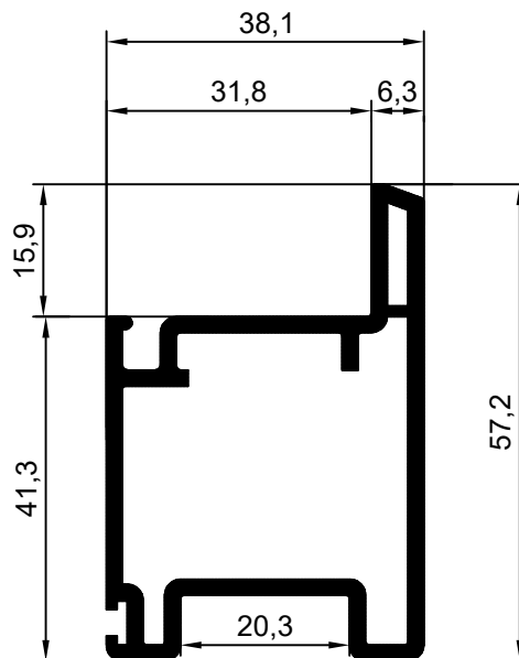
201603-231 Hoja común superior e inferior blanco 201603-233 Hoja común superior e inferior beige 201603-236 Hoja común superior e inferior clay
