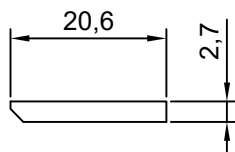
604368-301 Taco de acristalar S190
