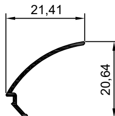
500012-231 Junquillo p/cristal senc. 3-6mm Blanco 500012-233 Junquillo p/cristal senc. 3-6mm Beige 500012-236 Junquillo p/cristal senc. 3-6mm Clay
