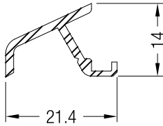
227848-001 Listón tope aluminio para puerta
