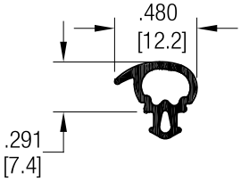
865960-001 Junta para Plegable 4500
