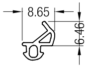
330101-001 Junta de hoja
