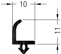
864940-010 Junta de batiente
