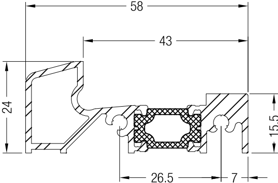
260000-004 Umbral aluminio para puerta
