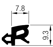
865022-001 Junta de acristalar No. 68
