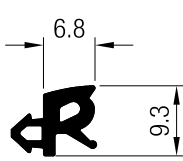
865012-001 Junta de acristalar No. 67
