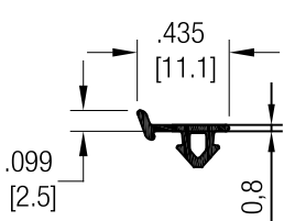
601575-001 Junta de acristalar No. 2.5
