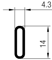
500093-002 Perfil de unión para marcos
