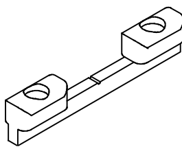
Liberadores de hoja
