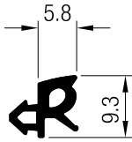
865002-010 Junta de acristalar No. 66
