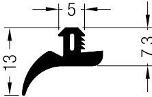
865070-002 Junta Inferior Pta de calle
