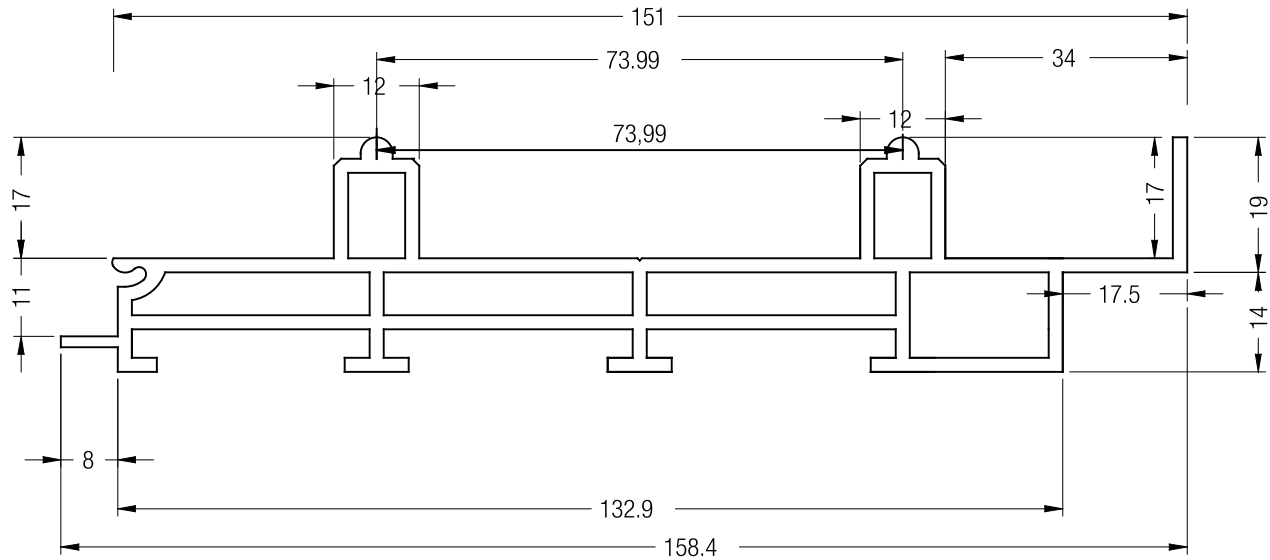
245565-001 Riel de aluminio encastrado S920-86
