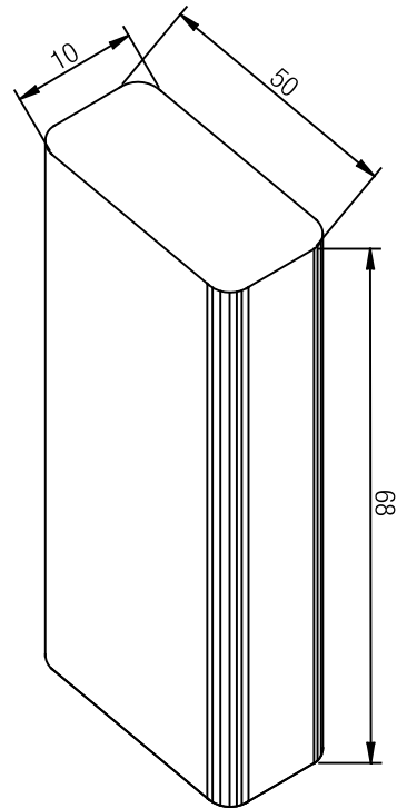
245567-001 Unión mecánica para guía encastada S920-86
