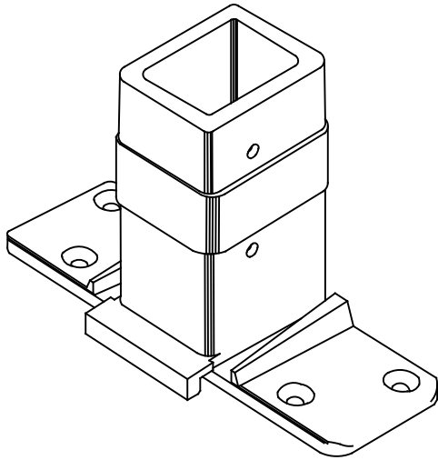
261758-001 Unión mecánica S920-86 para travesaño T86
