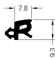
865022-001 Junta de acristalar No. 68
