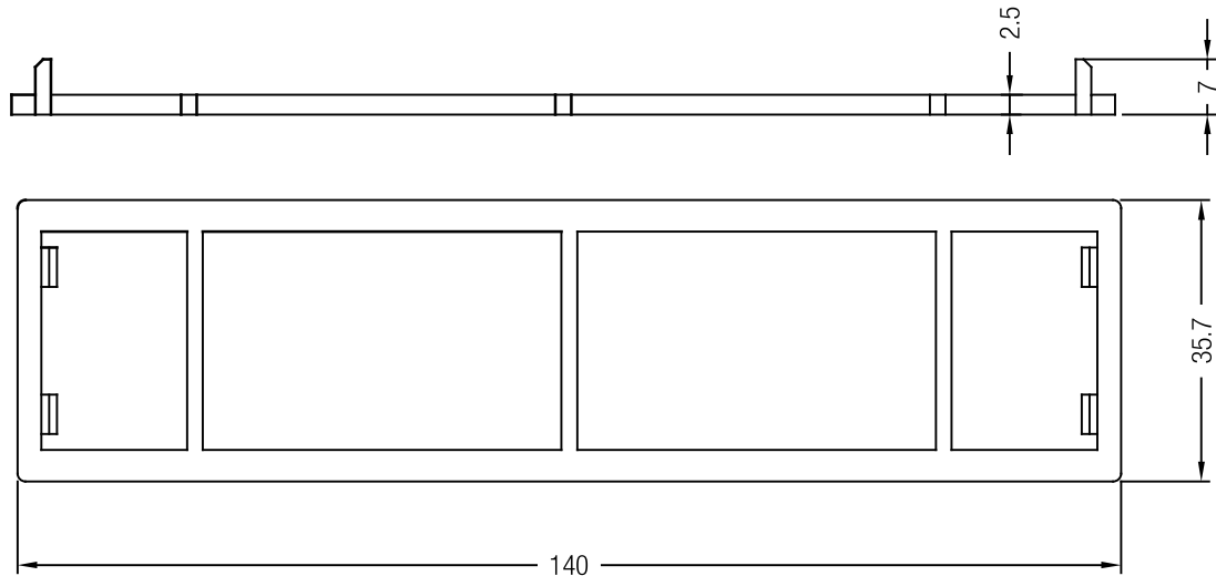
229294-002 Nivelador p/pza. de estanqueidad M3
