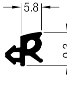
865002-010 Junta de acristalar No. 66
