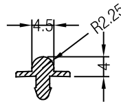
221842-001 Riel de aluminio S920
